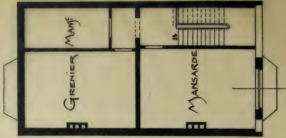
COMBLES.
